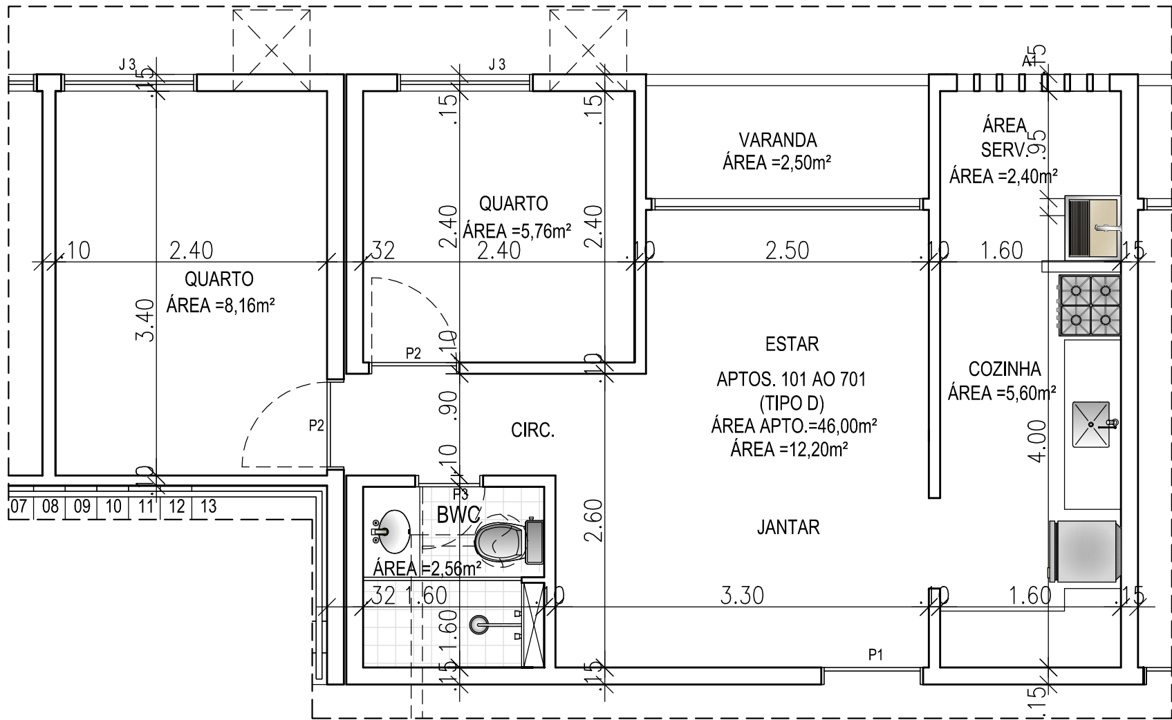
PAVTO. TIPO BLOCOS 01-02 APTO 01
