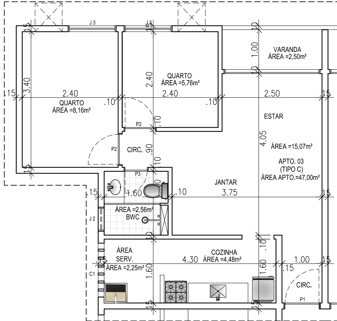
PAVTO. TÉRREO BLOCOS 04-05-07 APTO 03
