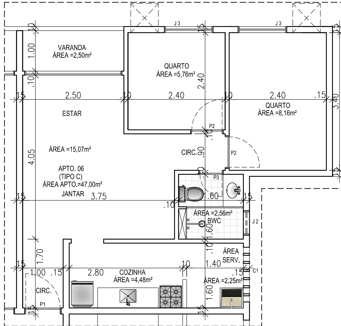
PAVTO. TÉRREO BLOCOS 04-05-07 APTO 06
