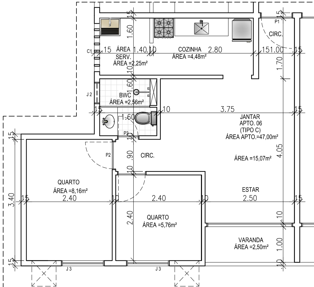
PAVTO. TÉRREO BLOCOS 01-02 APTO 06
