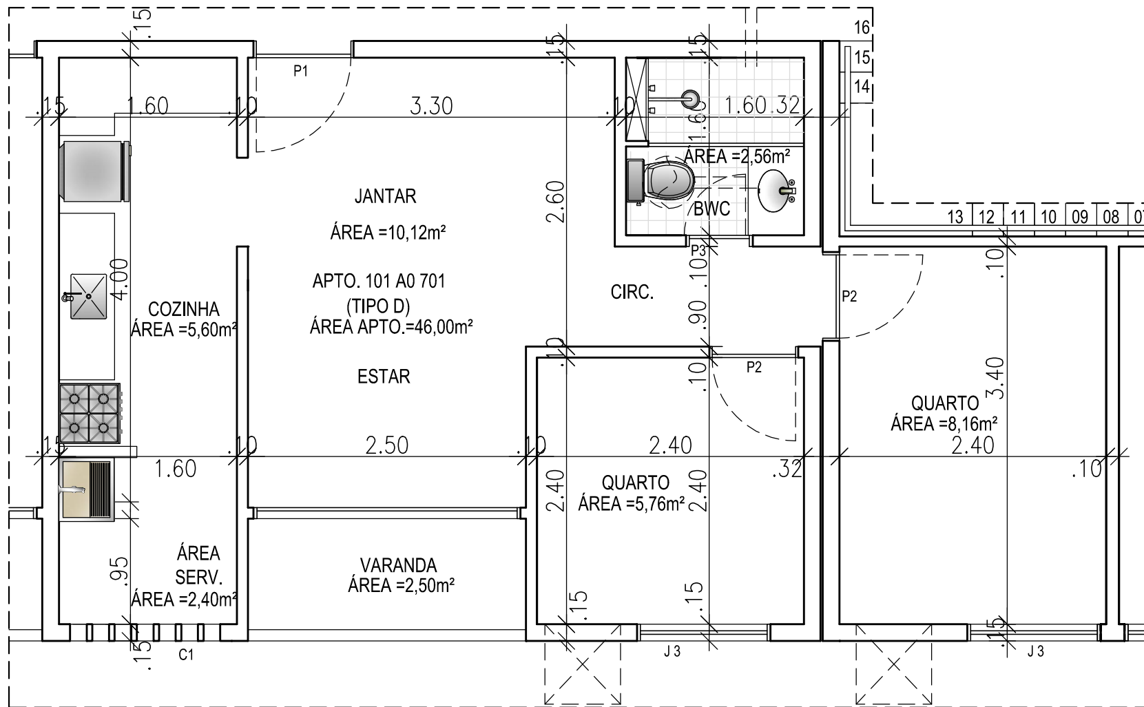
PAVTO. TIPO BLOCOS 04-05-07 APTO 01
