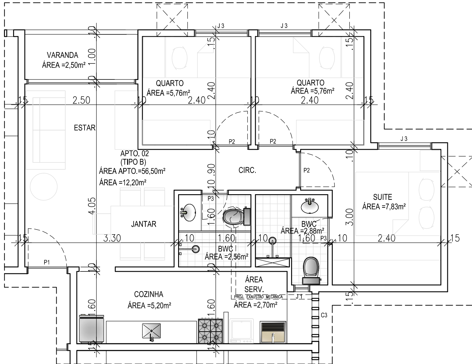
PAVTO. TÉRREO BLOCOS 01-02 APTO 02
